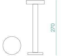
Ø90 Ø75 270
